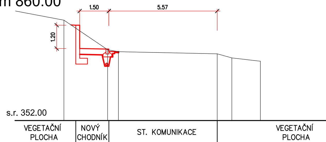
ŘEZ km 860.00
