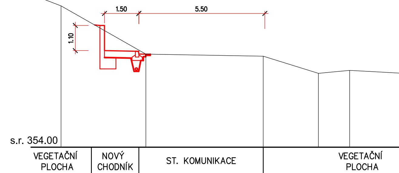
ŘEZ km 1 000.00 - variantní řešení
