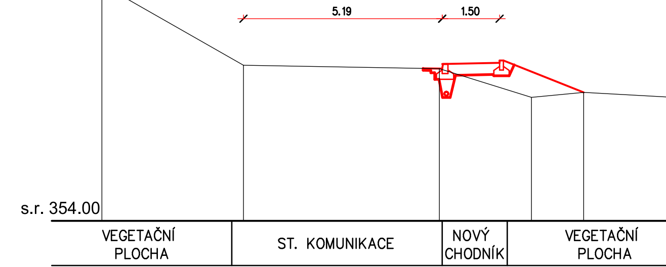
ŘEZ km 1 000.00
